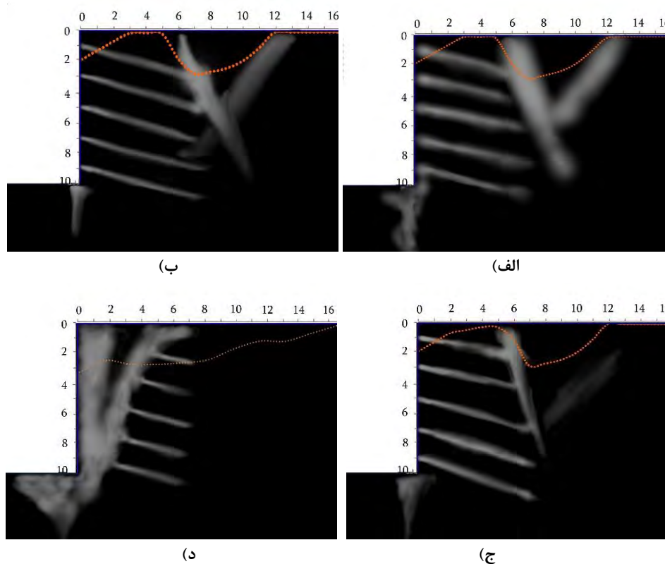
شکل ۱۶: سطوح گسیختگی در گوشه گود برای خاک ماسه‌ای؛ الف) گود مقعر با زاویه 60^\circ ، ب) گود مقعر با زاویه 90^\circ ، ج) گود مقعر با زاویه 120^\circ ، د) گود محدب با زاویه 27^\circ .
