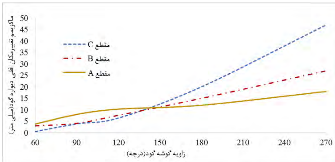
شکل ۱۴: نمودار ماکزیمم تغییرمکان افقی دیواره گود-زاویه گوشه برای خاک ماسه‌ای
