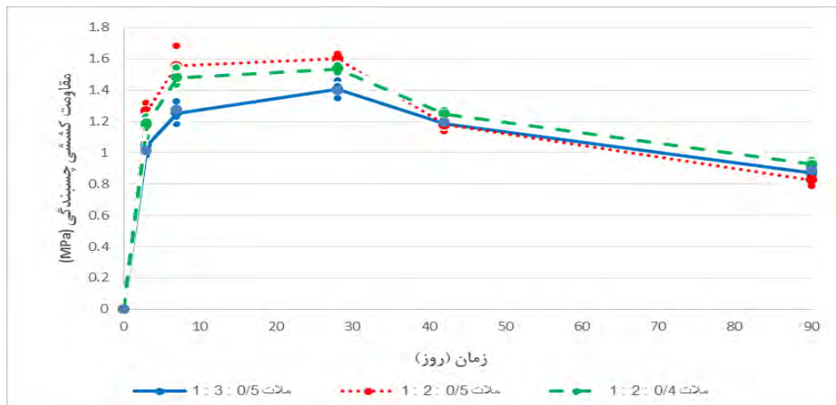
شکل ۱۰: مقاومت کششی چسبندگی حاصل از روش "کشش مستقیم" برای نمونه‌های عمل‌آوری ۷ روزه
