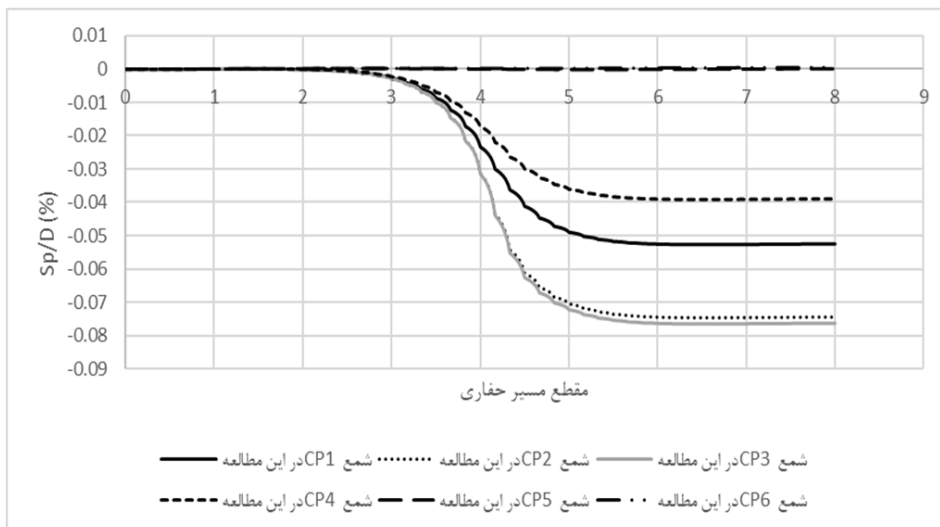
شکل ۷: خروجی نشست در طول تونل زنی مربوط به ۶ شمع در سه گروه شمع در تونلی با قطر ۱۱ متری
