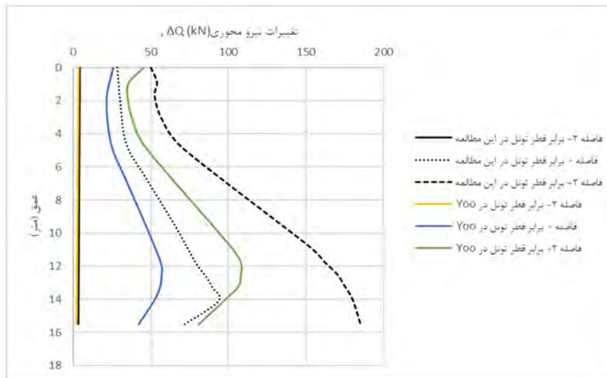
شکل ۲۴: تغییرات بار طول شمع CP3 در حین پیشروی تونل در فواصل مختلف
