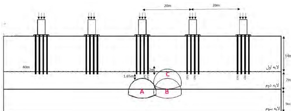
شکل ۲: محل احداث تونل زنی نسبت به نوک شمع
