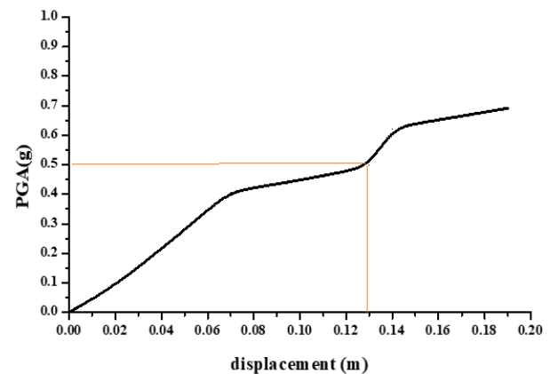
شکل ۸: منحنی دینامیکی فزاینده پل کابلی بیل امرسون تحت رکورد حوزه‌ی نزدیک گسل نورث ریج
