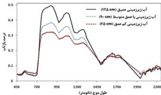
شکل ۵: بازتابندگی‌های طیفی گیاه نیشکر تحت مقادیر مختلف عمق آب زیرزمینی
