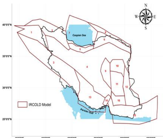
شکل ۱- مدل لرزه زمین ساختی کمیته ملی سدهای بزرگ ایران
