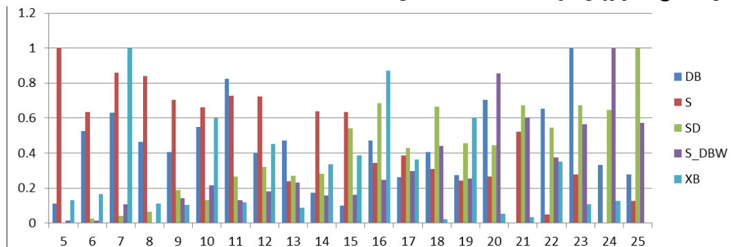
شکل ۳ - مقادیر شاخص های اعتبارسنجی روش کا-مینز از ۵ تا ۲۵ خوشه
