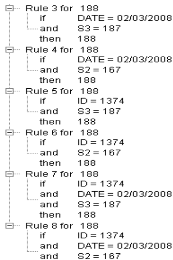
شکل ۹: تعدادی از قوانین استخراج شده از الگوریتم GRI
