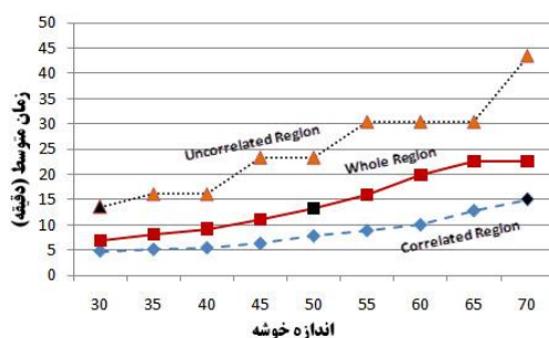
شکل ۱۱- نمودار زمان رسیدن کارشناس به محل حادثه با تغییر اندازه خوشه
