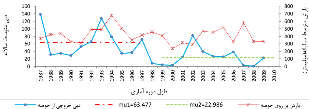
شکل ۵: نمودار متوسط دبی خروجی حوضه زربینه رود
