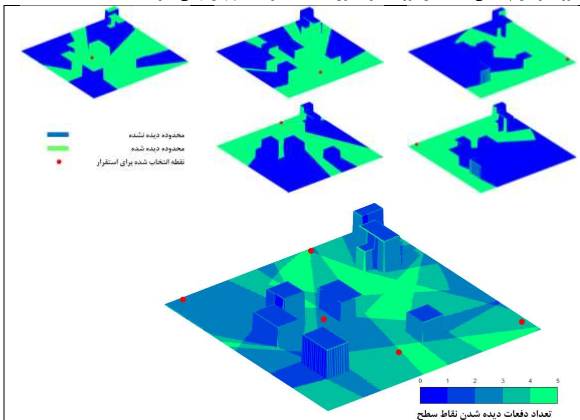
شکل ۸: وضعیت نقاط مختلف نهایی انتخاب شده برای پوشش کامل محدوده مورد نظر برای اسکن مربوط به نقاط انتخاب شده در شکل (۴)
