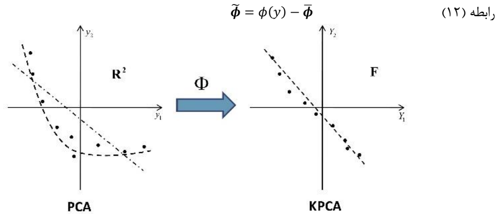
شکل ۲: ایده اصلی استفاده از KPCA با هسته کرنل غیرخطی [۲۳]
