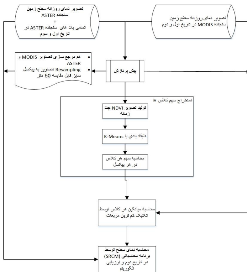
شکل ۱: طرح کلی الگوریتم STDEFA
