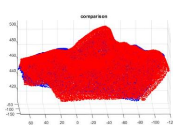
چهره ۵ - RMSE: 2.9616
