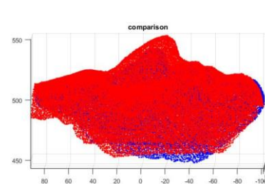
چهره ۲۵ - RMSE: 3.1541
