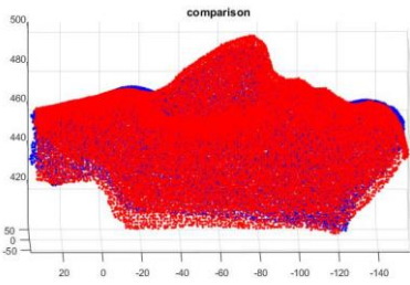
چهره ۴ - RMSE: 2.1447
