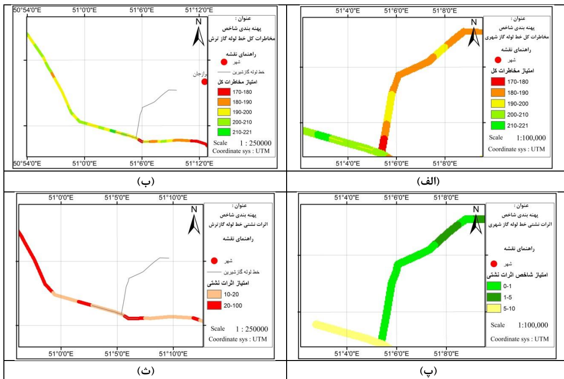
شکل ۷: (الف) نقشه پهنه بندی شاخص مخاطرات کل خط لوله گاز شهری، (ب) نقشه پهنه بندی شاخص مخاطرات کل خط لوله گاز ترش، (پ) نقشه پهنه بندی شاخص اثرات ناشی خط لوله گاز شهری، (ث) نقشه پهنه بندی شاخص اثرات ناشی خط لوله گاز ترش
