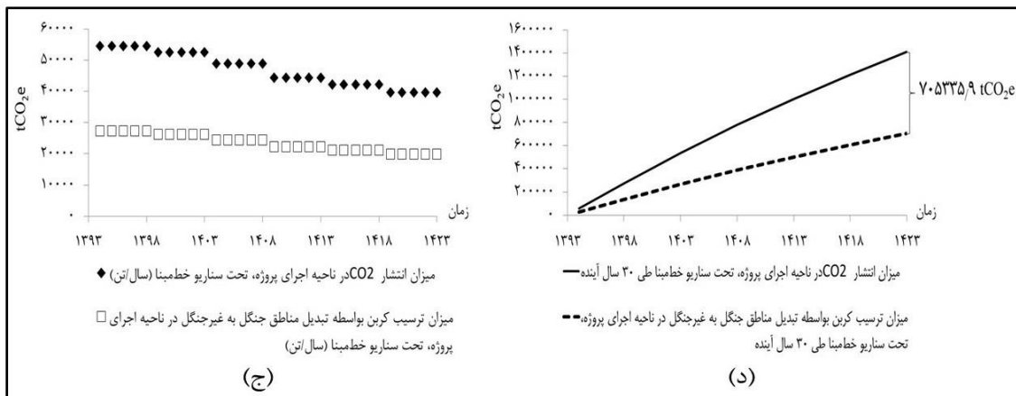
شکل ۱۱: (ج) میزان انتشار \text{CO}_2 و ترسیب کربن در ناحیه اجرای پروژه تحت سناریو خط مبنا، (د) نمودار تجمعی میزان انتشار \text{CO}_2 و ترسیب کربن در ناحیه اجرای پروژه تحت سناریو خط مبنا (طی ۳۰ سال آینده)
