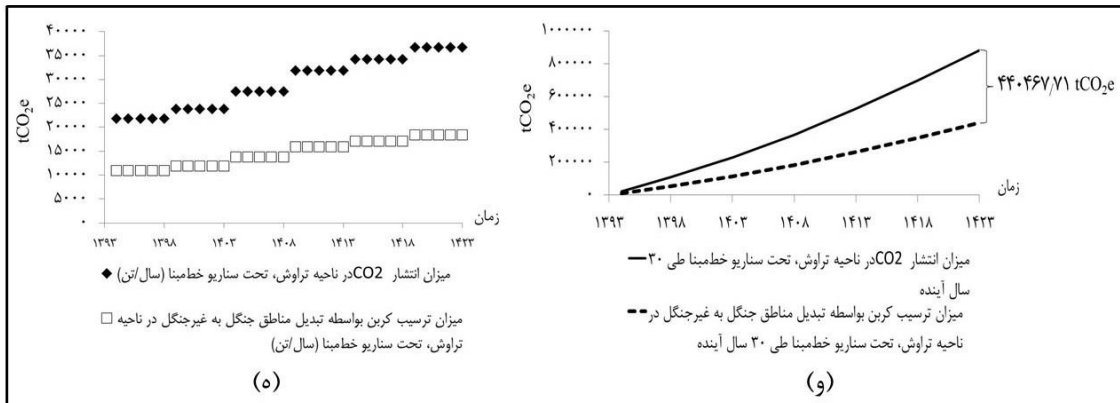
شکل ۱۲: (ه) میزان انتشار CO 2 و ترسیب کربن در ناحیه تراوش تحت سناریو خط‌مبنا، (و) نمودار تجمعی میزان انتشار CO 2 و ترسیب کربن در ناحیه تراوش تحت سناریو خط‌مبنا (طی ۳۰ سال آینده)
