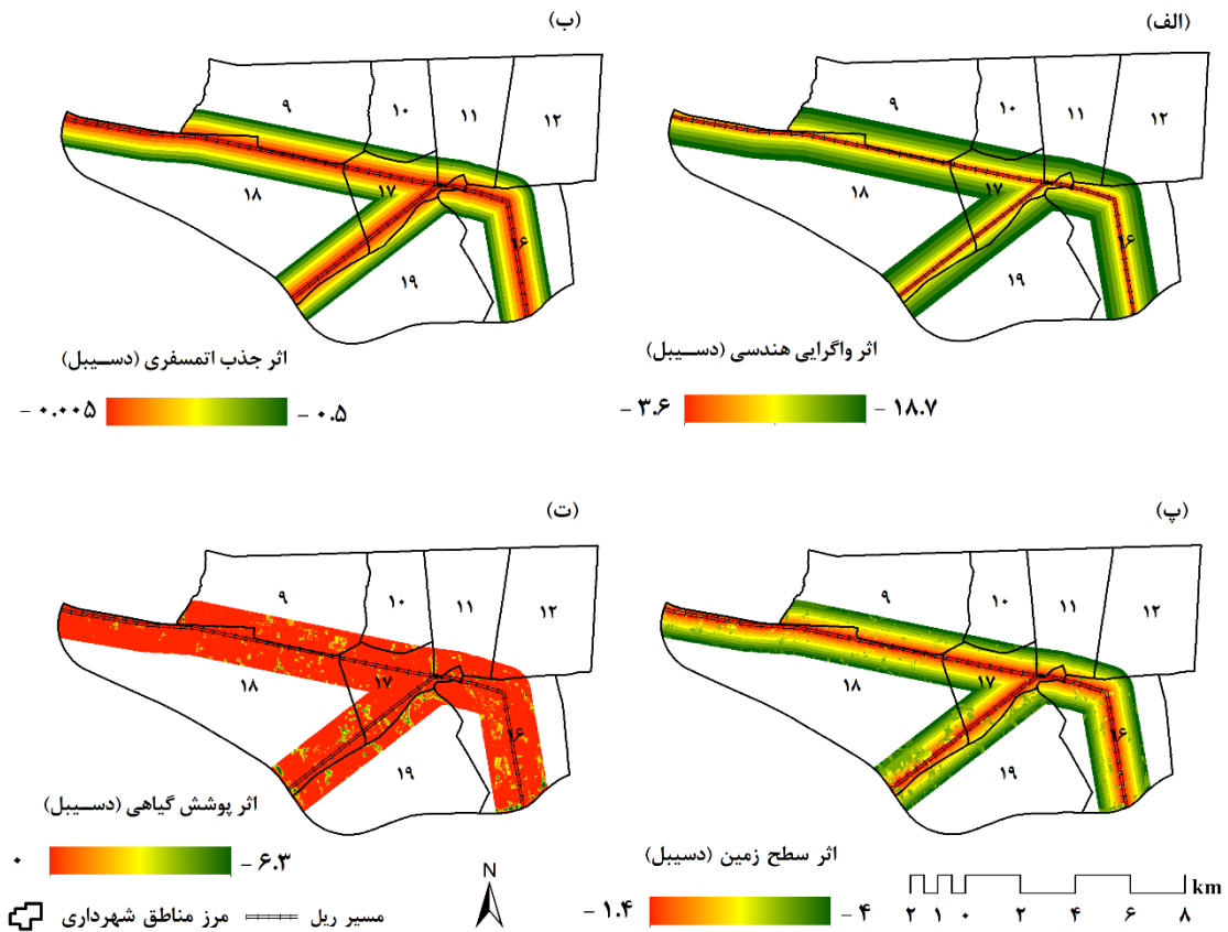
شکل ۲: عوامل تضعیف تراز صدا در محیط انتشار. الف) تضعیف ناشی از واگرایی هندسی (افزایش فاصله از منبع)، ب) تضعیف ناشی از جذب اتمسفری، پ) تضعیف ناشی از اثر سطح زمین، ت) تضعیف ناشی از جذب پوشش زمین (پوشش گیاهی)
