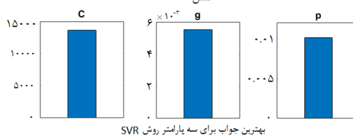
ج- نمودار بهینه‌سازی پارامترهای SVR برای تصویر سنیتیل ۲
