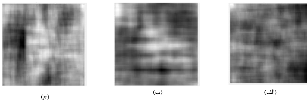
شکل ۷: خروجی حاصل از اعمال برخی از فیلترهای کانولوشن بر روی داده‌های آموزشی تبدیل شده به قطعات ۲۹ در ۲۹ (الف) نقشه ویژگی اول، (ب) نقشه ویژگی دهم، (ج) نقشه ویژگی بیستم)
