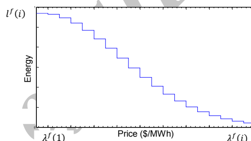
شکل ۳: نمودار چندپله ای قیمت برق-انرژی مسئله خرده فروش
