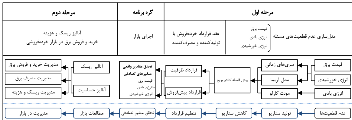
شکل ۲: مراحل برنامه‌ریزی تصادفی در بهینه‌سازی سبد انرژی
