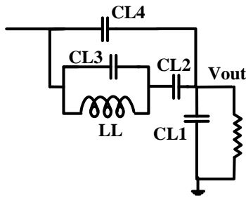
شکل ۷: فیلتر خروجی طبقات
