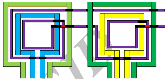
شکل ۶: چیدمان پیشنهادی مدار ترکیب کننده توان
