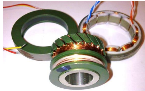
شکل ۳: استاتور و رتور ریزالور مورد مطالعه به همراه اولیه و ثانویه ترانسفورماتور گردان (نمونه عملی ساخته شده)
