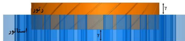
شکل ۷: ریزالور مورد مطالعه تحت خطای رانش محوری به اندازه \gamma
