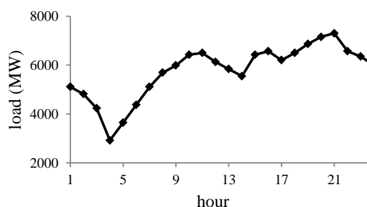
شکل ۶: پروفایل بار روزانه سیستم مورد مطالعه
