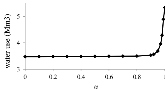
شکل ۹: آب مصرفی سیستم بر حسب مقادیر مختلف ضریب \alpha
