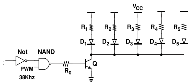
شکل ۲: مدار فرستنده
