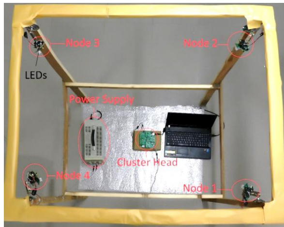
شکل ۵: ساختار شبکه طراحی شده. چهار گره و یک سرخوشه
