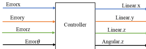
شکل ۵: ورودی‌ها و خروجی‌های کنترلر خارجی
