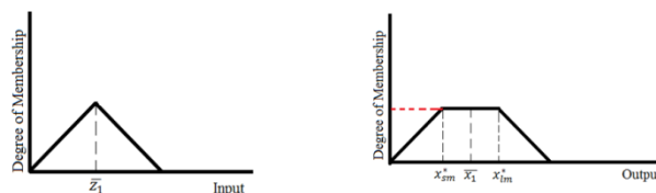
شکل ۱۳: تابع عضویت خروجی قطع شده با درصد عضویت و طول مرکز سطح نمودار \bar{x}_1 و خروجی نهایی x_{lm}^* برای روش بزرگ ترین بیشینه و خروجی نهایی x_{sm}^* برای کوچک ترین بیشینه (راست). تابع عضویت ورودی با طول مرکز مساحت زیر نمودار \bar{z}_1 (چپ)
