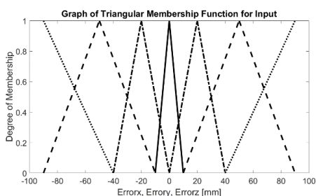
شکل ۶: تابع عضویت مثلثی برای ورودی‌ها، مجموعه‌ها توسط شکل خطوط
