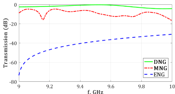
شکل ۱۰- بررسی اثر به کارگیری فرا ماده در تغییردهنده فاز
