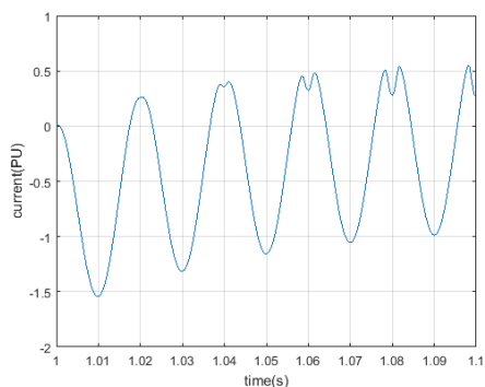
ج- جریان دیفرانسیل فاز a در شرایط خطای خارجی سه فاز
