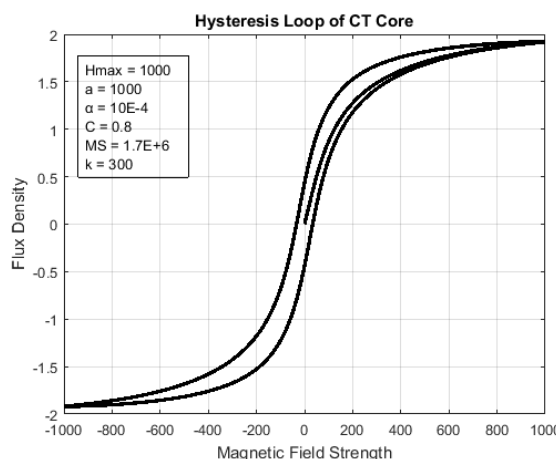
شکل ۳: حلقه هیستریزیس هسته ترانسفورماتور جریان
