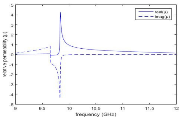
شکل ۶: مقادیر حقیقی و موهومی ضریب نفوذ پذیری مغناطیسی نسبی سلول فرامواد
