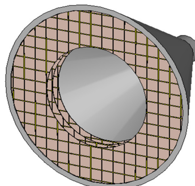
شکل ۹: نمایش سه بعدی آنتن شیپوری مخروطی با طول ۱۵۶.۸۴۹ میلی‌متر در حضور لنزهای فرامواد
