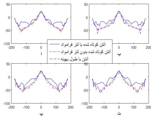
شکل ۱۱: الگوی تشعشی آنتن در زاویه سمت \varphi = 0^\circ و در فرکانس ۹ گیگاهرتز (ب) ۱۰ گیگاهرتز (پ) ۱۱ گیگاهرتز (ت) ۱۲ گیگاهرتز
