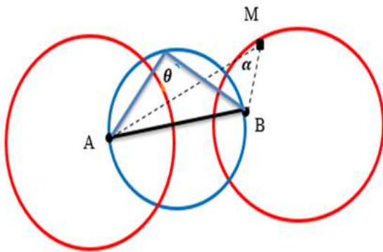
شکل ۳: دایره‌ی آپولونیوس و کمان درخور
