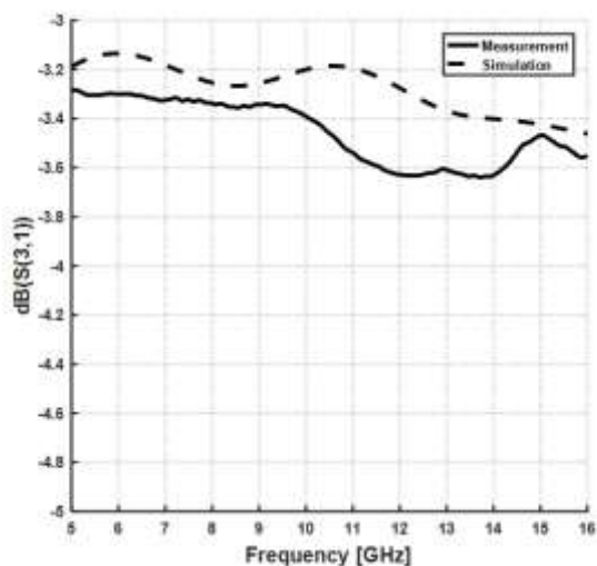
شکل ۱۴: نتایج حاصل از تست و شبیه‌سازی افت عبوری دهانه‌ی سوم تقسیم‌کننده‌ی توان فرایه‌ن‌باند
