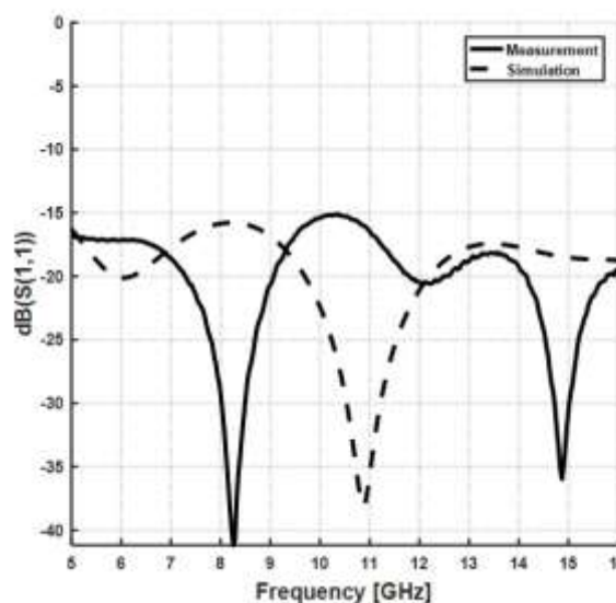
شکل ۱۲: نتایج حاصل از تست و شبیه‌سازی افت بازگشتی دهانه‌ی ورودی تقسیم‌کننده‌ی توان فرایه‌ن‌باند
