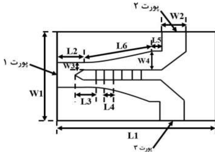
شکل ۹: تقسیم‌کننده‌ی توان طراحی‌شده در نرم افزار HFSS در ابعاد L_1=3\text{mm} ، L_2=5\text{mm} ، L_3=4/5\text{mm} ، L_4=2/7\text{mm} ، L_5=1\text{mm} ، L_6=14\text{mm} ، W_1=6/4\text{mm} ، W_2=2/3\text{mm} ، W_3=1/4\text{mm} ، W_4=8/75\text{mm} ،
