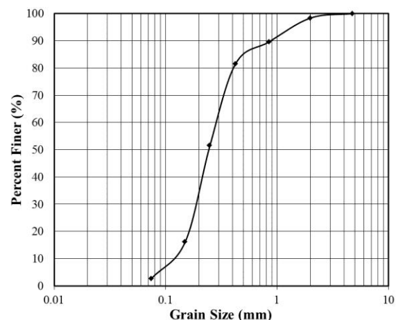
شکل ۱- منحنی دانه‌بندی خاک مورد استفاده
