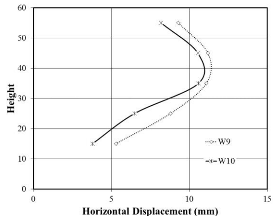
شکل ۱۲- تاثیر مهار تسلیح‌کننده بر تغییرشکل رویه در سربار ۱۲۰ kPa
