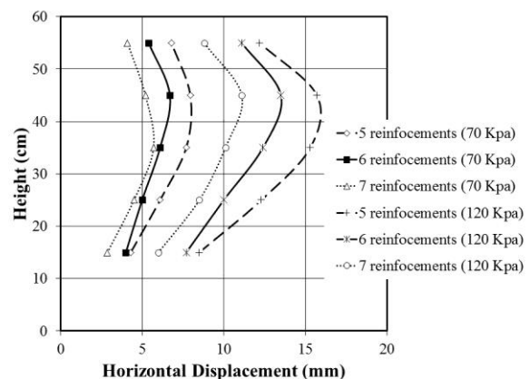
شکل ۳- تاثیر تعداد لایه تسلیح بر تغییرشکل افقی رویه
