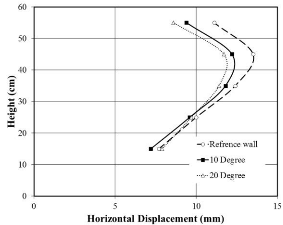
شکل ۹- تاثیر شیب تسلیح‌کننده‌ها بر تغییرشکل افقی در سربار ۱۲۰ kPa
