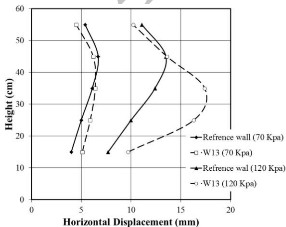
شکل ۱۱- تاثیر نزدیکی مهار به ناحیه گسیختگی رانکین بر تغییرشکل افقی
