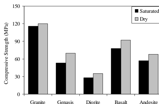
شکل (۱۴) مقاومت تک‌محوری (سنگدانه‌های آذرین)
