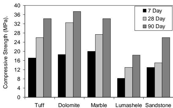
شکل (۱۶) مقاومت بتن ساخته شده (سنگدانه رسوبی و دگرگونی)
