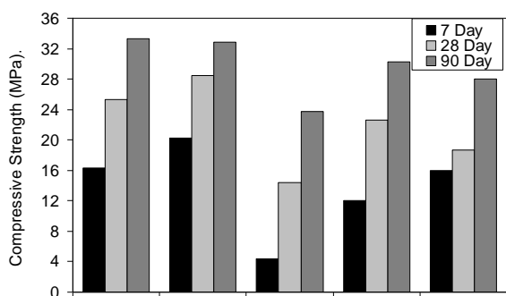
شکل (۱۷) مقاومت بتن ساخته شده (سنگدانه آذرین)
