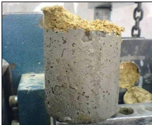
شکل (۱۰) نمونه لوماشل بعد از آزمایش
