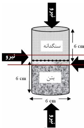
شکل (۲) تصویر شماتیک نمونه آزمایش شده
