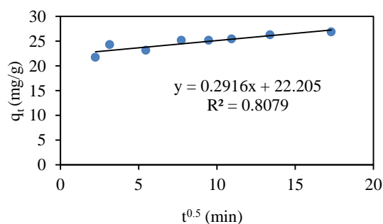
شکل (۱۰) مدل نفوذ درون‌ذره‌ای برای جذب MB روی PS (۳/۵ mg/l) در pH=۷
