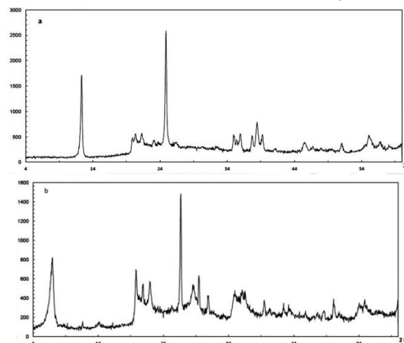
Fig. 1. XRD spectrum a- Kaolinite b- Bentonite
