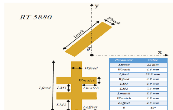
شکل (۳): نمای شبکه تغذیه (پشت آنتن) آنتن طراحی شده.
