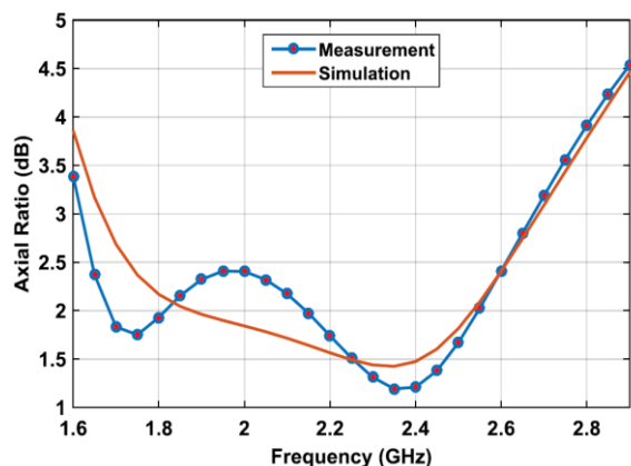
شکل (۷): منحنی AR آنتن.
