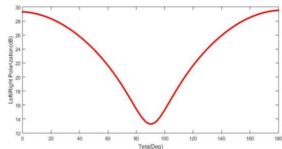
شکل (۱۲): نسبت قطبش چپ گرد و راستگرد.
