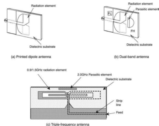
شکل (۱): چند نمونه آنتن ایستگاه‌های پایه [۸].
