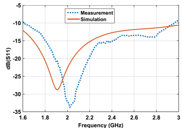
شکل (۶): منحنی S_{11} آنتن.
