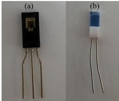
شکل (۴): نمای ظاهری مازول حسگر رطوبت (a) و دمای هوا (b).
