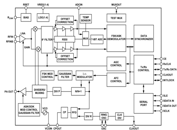
شکل (۵): شمای کلی فرستنده ADF7020.
