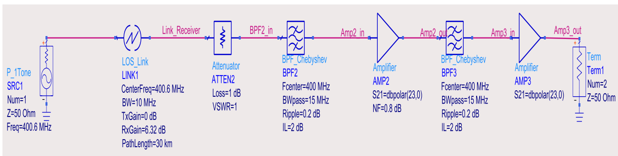
شکل (۱۶): مسیر مخابراتی شبیه سازی گیرنده زمینی.
