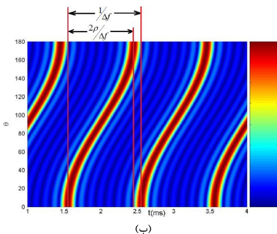
شکل (۲): الگوی تشعشعی آرایه FDA خطی (الف) نمایش سه‌بعدی (ب) نمایش دوبعدی زمان-زاویه
