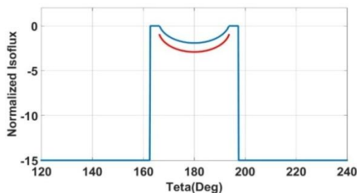
شکل (۱۰): ماسک پرتو تشعشعی زینی شکل برای سنتز مرز بالا و پایین زینی شکل.
