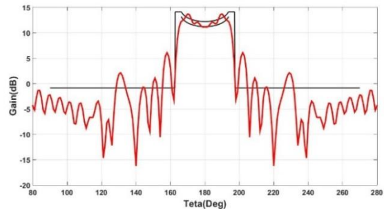
شکل (۱۴): نمای پرتو دوبعدی سنتز شده زینی شکل در باند X @ 5/8 GHz با تعداد ۲۲×۲۲ المان سلول واحد.
