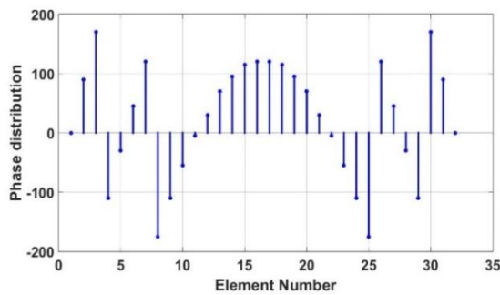
شکل (۹): فاز مطلوب بیم زینی شکل برای نقطه شروع اولیه سنتز.
