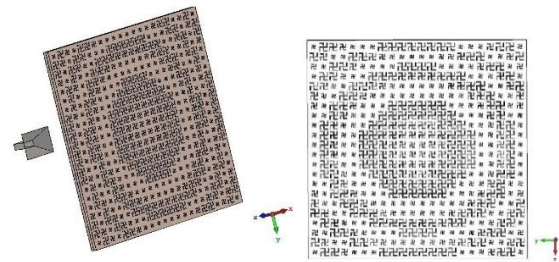
شکل (۱۳): شکل نمای کلی آنتن ارائه انتقالی برای سنتز پرتو زینی شکل با تعداد عناصر ۲۲×۲۲ و فاصله‌گذاری F/D=0.8 .
