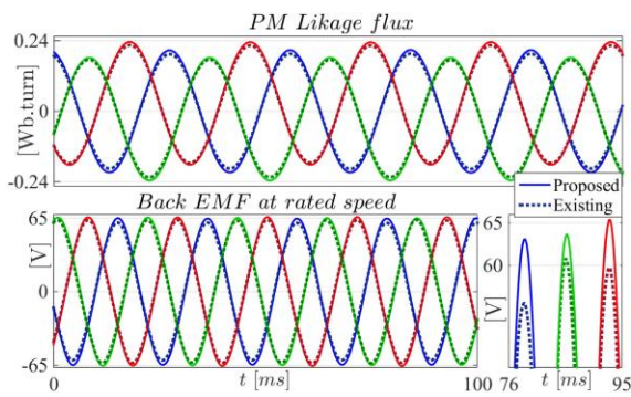
شکل (۳): شار پیوندی و ولتاژ بی باری ماشین.
