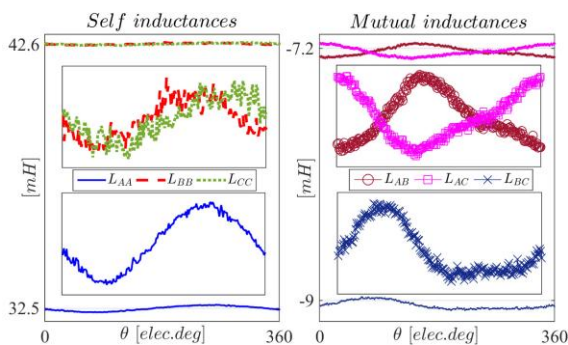
شکل (۴): اندوکتانس خودی و متقابل فازهای ماشین.
