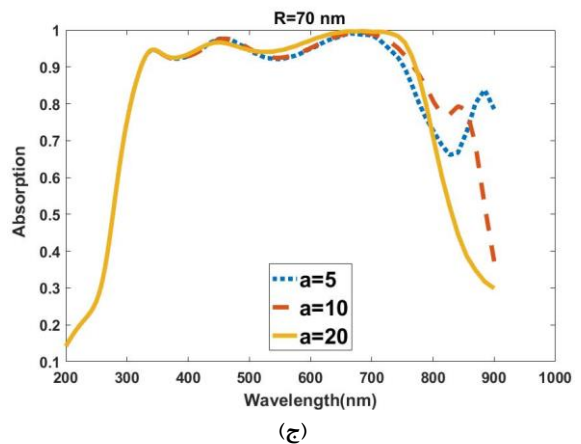
شکل (۵): منحنی جذب به ازای فواصل ۵، ۱۰ و ۲۰ نانومتر نانوذرات از هم در شعاع نانوذرات (الف) ۲۵ nm، (ب) ۵۰ nm و (ج) ۷۰ nm.
