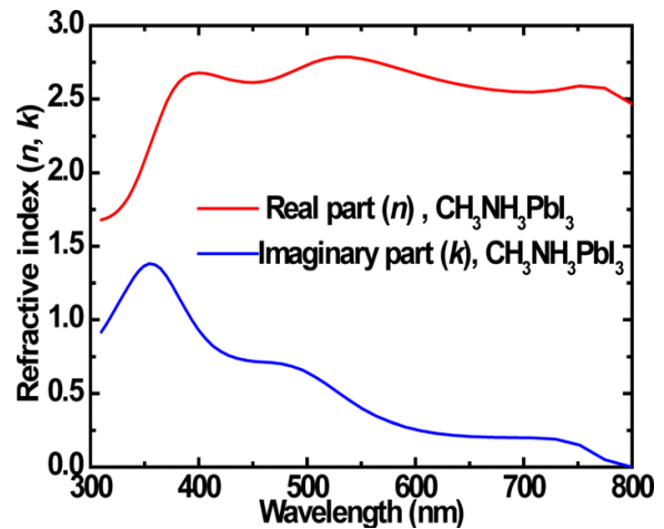
شکل (۲): منحنی ضریب شکست و ضریب خاموشی ماده CH_3NH_3PbI_3 [۴۰].
