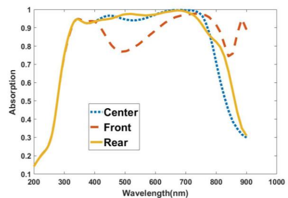
شکل (۷): منحنی جذب به ازای موقعیت‌های مختلف نانوذرات در جلو، عقب و وسط لایه پروسکایت.
