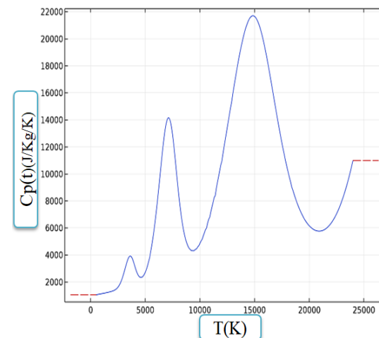
شکل (۳): ظرفیت گرمایی هوا Cp وابسته به دما
