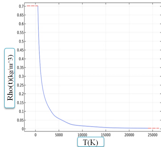
شکل (۲): چگالی هوا وابسته به دما
