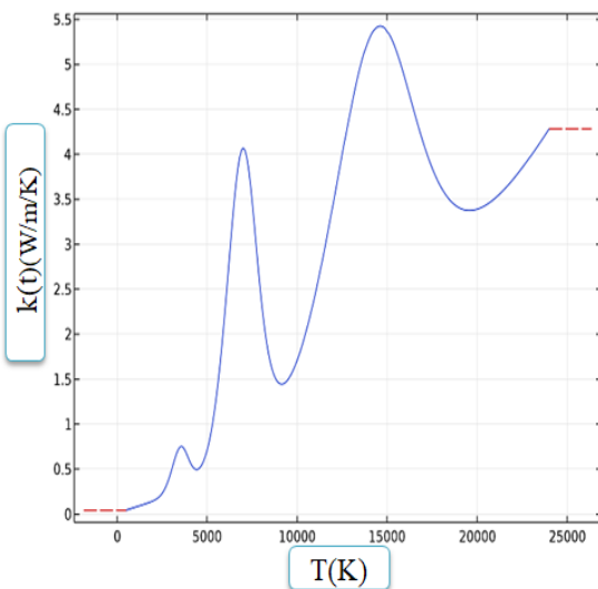
شکل (۵): هدایت حرارتی هوا وابسته به دما
