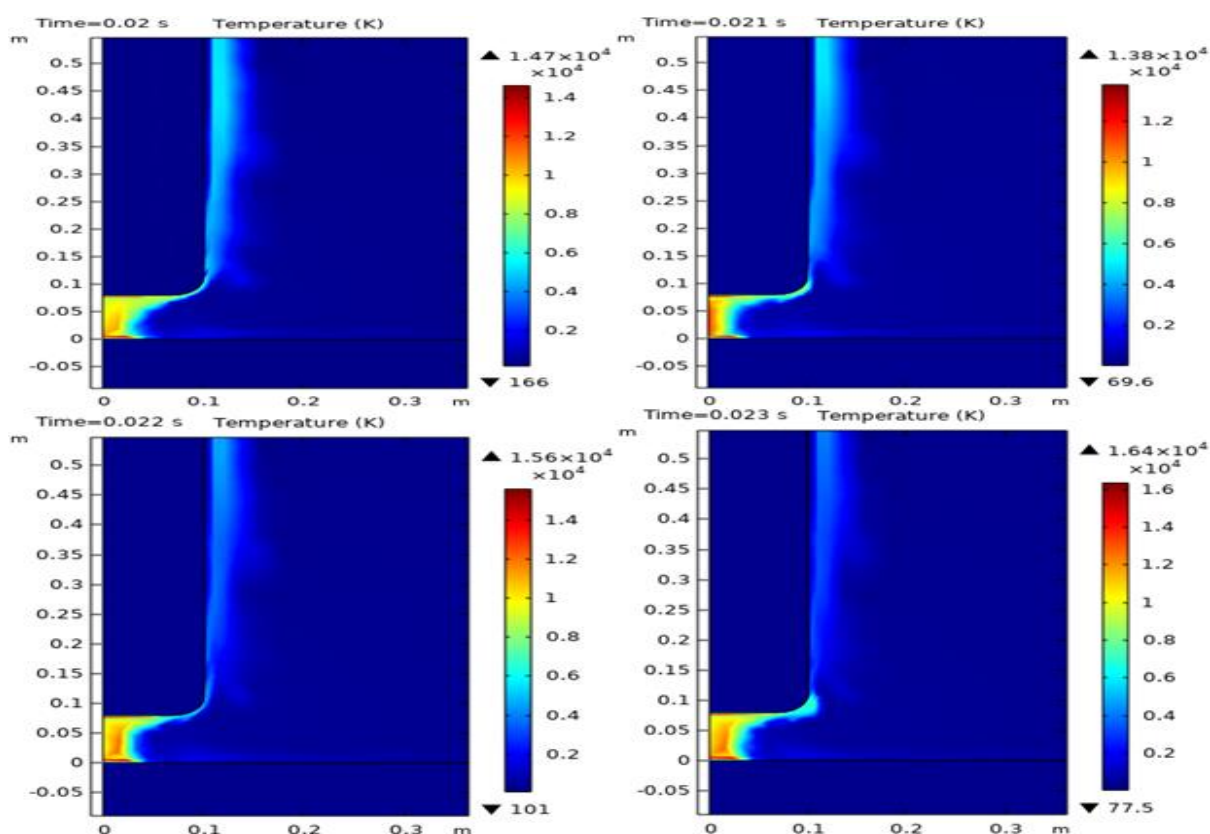
شکل (۱۵): دمای ستون قوس الکتریکی بر حسب (K) در زمان‌های ۰/۰۲، ۰/۰۲۱، ۰/۰۲۲ و ۰/۰۲۳ ثانیه
