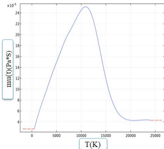
شکل (۴): گرانیوی دینامیکی هوا وابسته به دما
