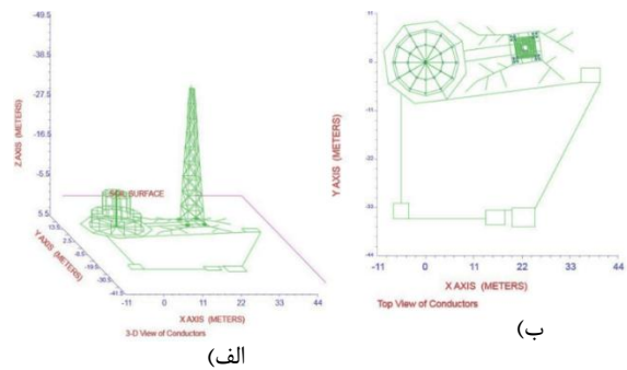
شکل (۱۲): آرایش درختی سامانه زمین سایت بمو، (الف) نمای سه‌بعدی (ب) نمای از بالا
