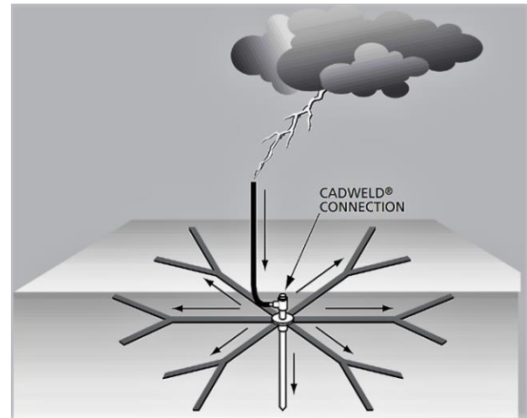
شکل (۱۱): آرایش درختی الکترودهای زمین [۲۵].
