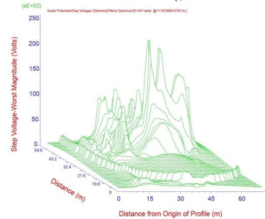
شکل (۱۸): الف) ولتاژ گام ب) ولتاژ تماس در روش شعاعی
