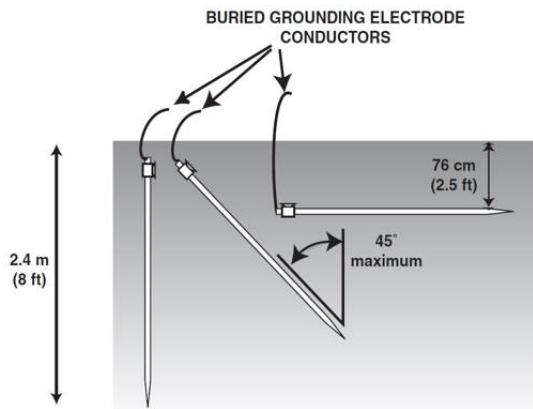
شکل (۸): زاویه دفن میله‌ها در زمین [۲۱]
