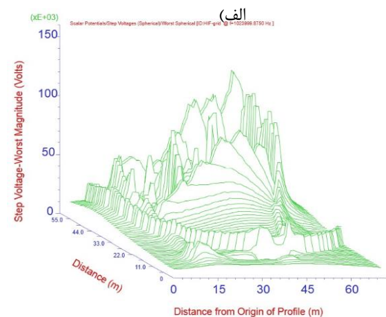
شکل (۲۲): (الف) ولتاژ گام (ب) ولتاژ تماس در روش مش
