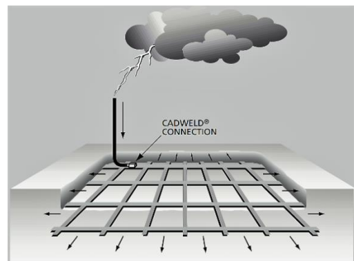
شکل (۱۹): آرایش مش الکترودهای زمین [۲۵].
