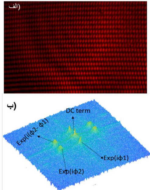
شکل (۳): (الف) طرح تداخلی باریکه‌های بازگشتی از لیزر (ب) تبدیل فوریه این طرح تداخلی و قله‌های مربوط به اطلاعات دو وجه
