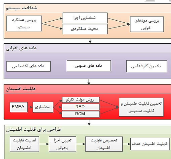
شکل ۴. روند ارائه‌شده برای ارزیابی و طراحی قابلیت اطمینان سیستم
