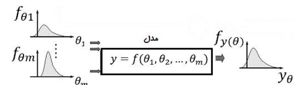
شکل ۳. نمایی از فرایند شبیه‌سازی مونت کارلو [۱۴]
