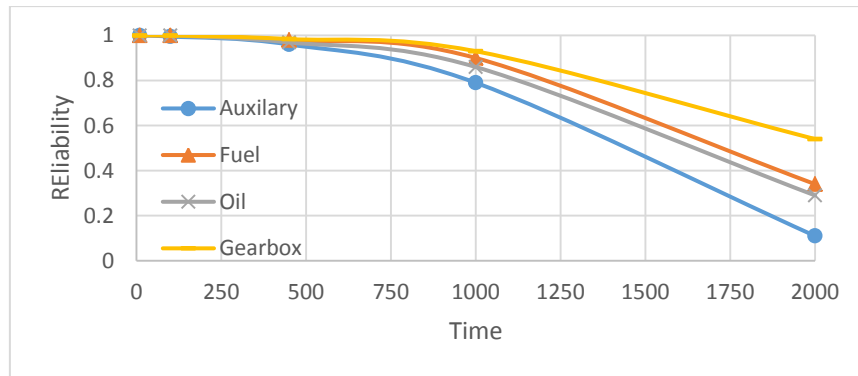
شکل ۱۸. تغییرات قابلیت اطمینان اجزای زیرسیستم کمکی بر حسب زمان
