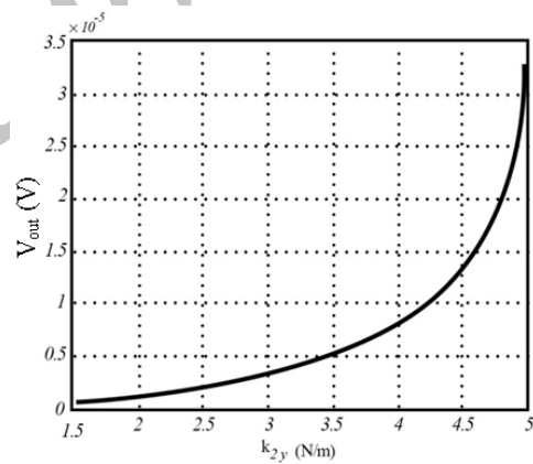
شکل ۷. تغییرات ولتاژ خروجی سیستم نسبت به تغییرات سختی
