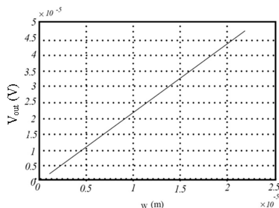
شکل ۹. تغییرات ولتاژ خروجی با تغییرات عرض ساختار
