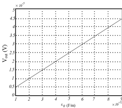
شکل ۸. تغییرات ولتاژ خروجی نسبت به تغییرات ضریب گذردهی
