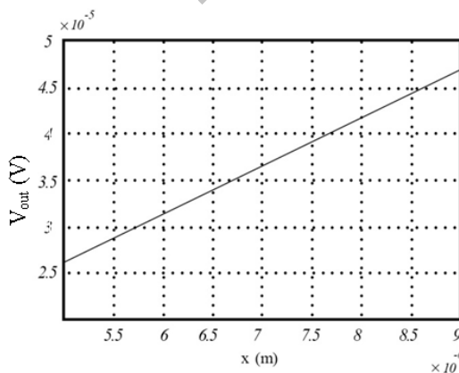
شکل ۱۰. تغییرات ولتاژ خروجی سیستم نسبت به تغییر طول ساختار
