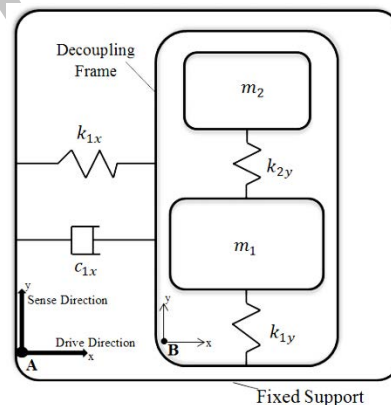
شکل ۲. مدل المان‌های متمرکز ساختار مکانیکی
