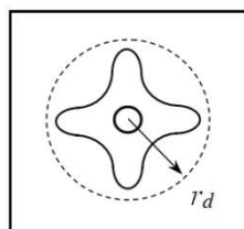
شکل ۵. شماتیک ناحیه لایه‌لایه شدن
