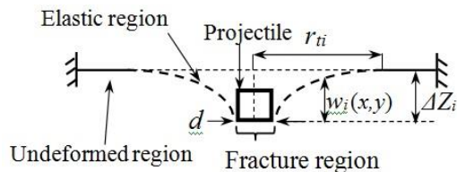
شکل ۲. شماتیک ورق؛ الف) قبل از برخورد، ب) بعد از برخورد
