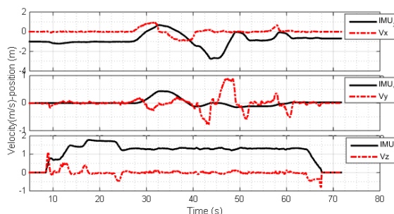
شکل ۱۷. تخمین موقعیت و سرعت با استفاده از حسگر اینرسیایی
