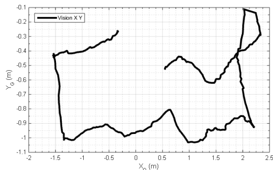
شکل ۱۵. نمودار تخمین موقعیت در هنگام حرکت دستی پرنده
