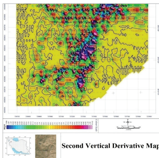
شکل ۶: نقشه مشتق قائم میدان مغناطیسی محدوده کرکرا
