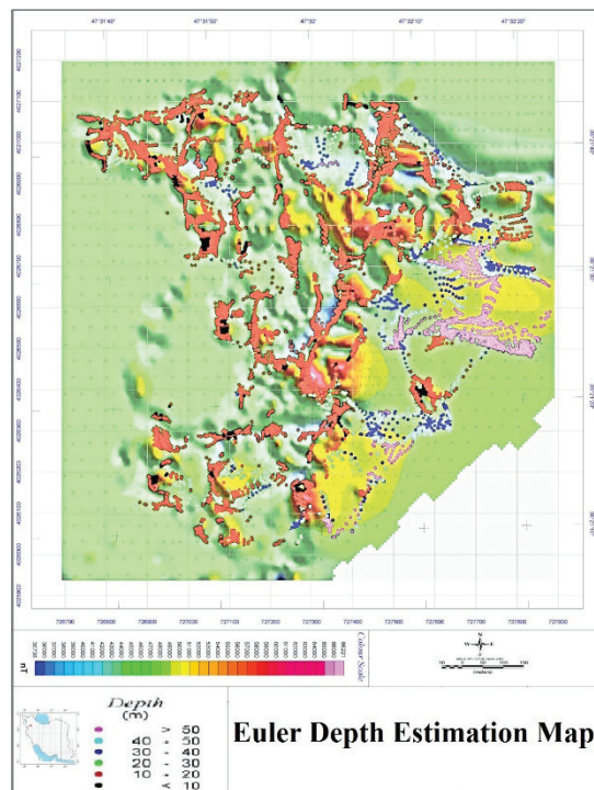
شکل ۱۲: نقشه تعیین عمق اویلر در منطقه کرکرا یک
