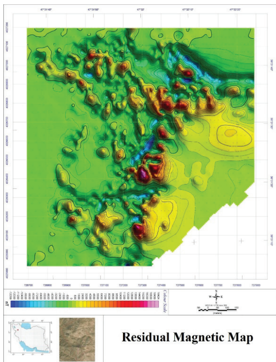
شکل ۵: نقشه شدت میدان باقیمانده در محدوده کرکرا یک
