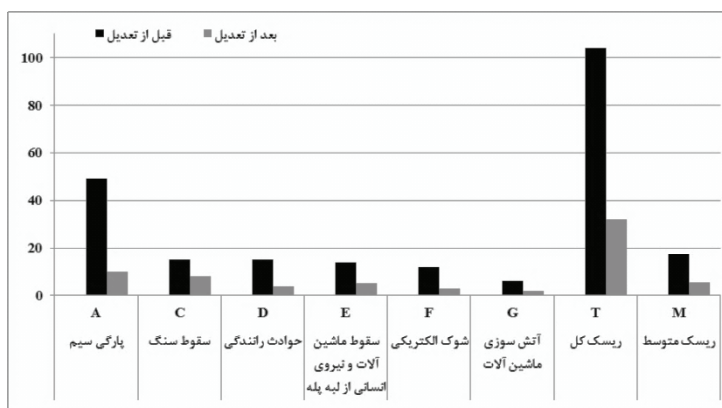
شکل ۳: نمودار مقایسه ریسک حوادث قبل و بعد از تعدیل
