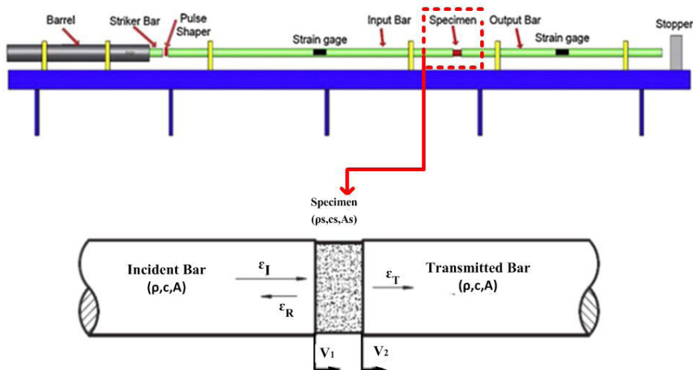
شکل ۸: نمای شماتیک دستگاه میله فشاری هاپکینسون
