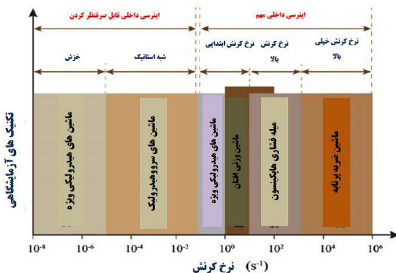
شکل ۷: تکنیک‌های اصلی بارگذاری برای تعیین خصوصیات مکانیکی مصالح در گستره نرخ
