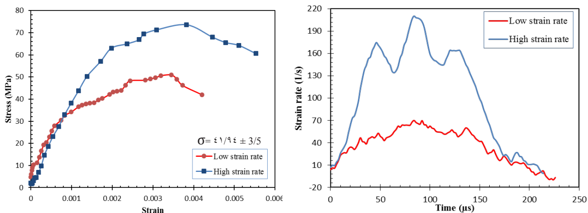
شکل ۱۰: رفتار دینامیکی مرمیت‌های مارون در نرخ کرنش پایین و بالا
