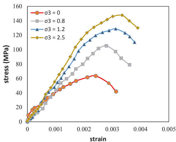
شکل ۱۳: منحنی تنش - کرنش مرمیت‌های مارون در بارگذاری شبه استاتیکی (چپ) و دینامیکی (راست)
