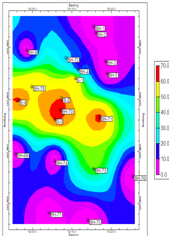
شکل ۳: نقشه موقعیت گمانه‌ها و نحوه توزیع عیار آهن در محدوده مورد مطالعه
